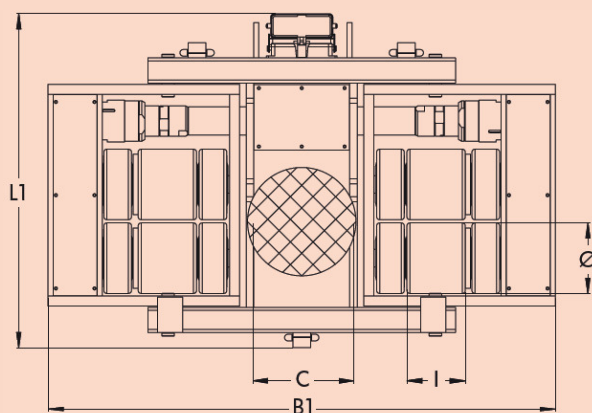
Vázlat JLA 15/30 G
