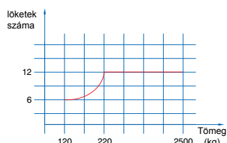
Quick-lift szivattyú diagram
